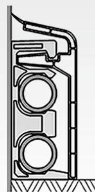
Řez zalištovaným potrubím
